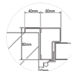
Profielafmeting
